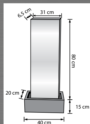
Muro II Art.-Nr.: 23009 Korpus: L31 x B6,5 x H80 cm Becken: L40 x B20 x H15 cm
