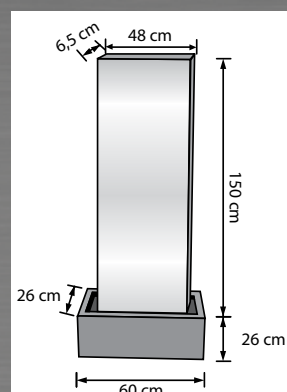
Muro I Art.-Nr.: 23008 Korpus: L48 x B6,5 x H150 cm Becken: L60 x B26 x H26 cm
